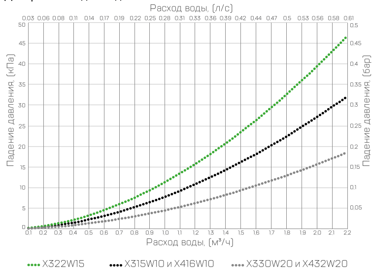
Диаграмма падения давления на теплообменниках X300W и X400W
