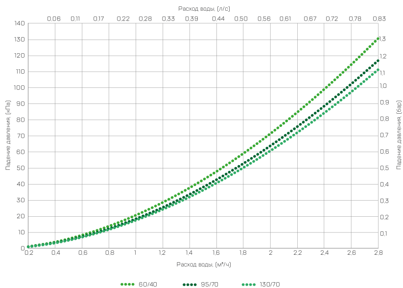
Диаграмма падения давления на теплообменнике тепловентилятора AERO15D30
