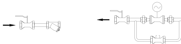
Смесительный узел с двухходовым клапаном без насоса
