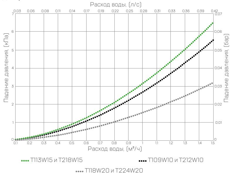
Диаграмма падения давления на теплообменниках T100W и T200W
