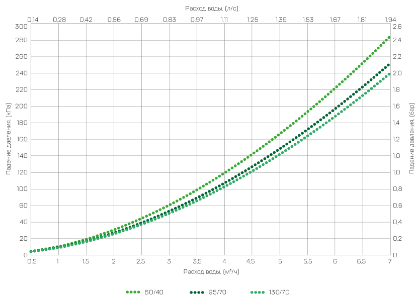
Диаграмма падения давления на теплообменнике тепловентилятора AERO 70D55
