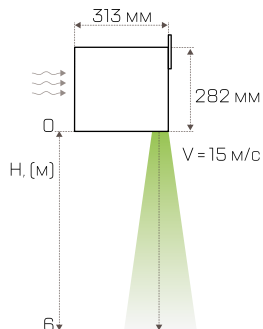
Габаритные размеры и характеристики потока
