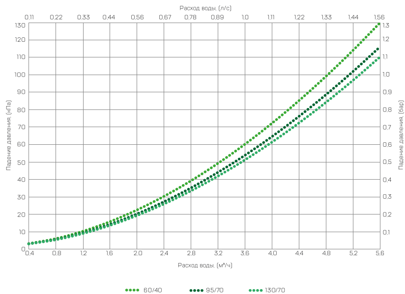
Диаграмма падения давления на теплообменнике тепловентилятора AERO 45D45
