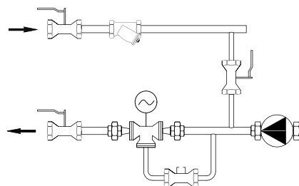
Смесительный узел с трехходовым клапаном с насосом
