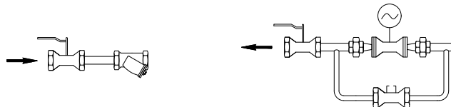
Смесительный узел с двухходовым клапаном без насоса
