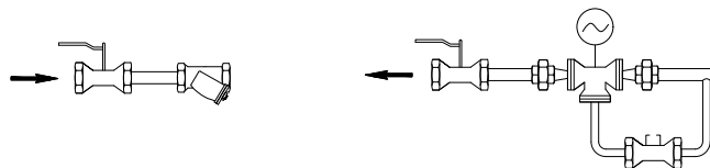
Смесительный узел с трехходовым клапаном с насосом
