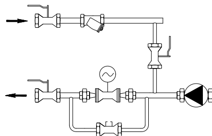
Смесительный узел с двухходовым клапаном с насосом
